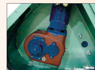
Moto-réducteur : Entraînement par moteur hydraulique et boîtier réducteur.
