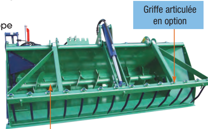
Vis à pas tronqué
