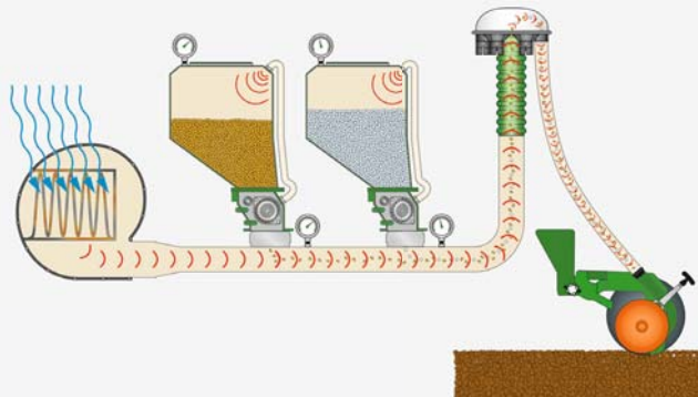
Principe du Cirrus-C
