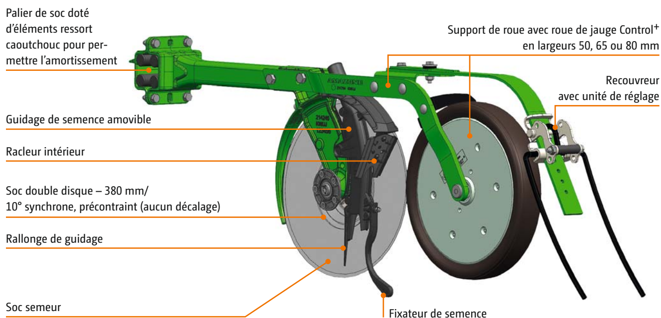
Double disque TwinTeC + (coupe)
